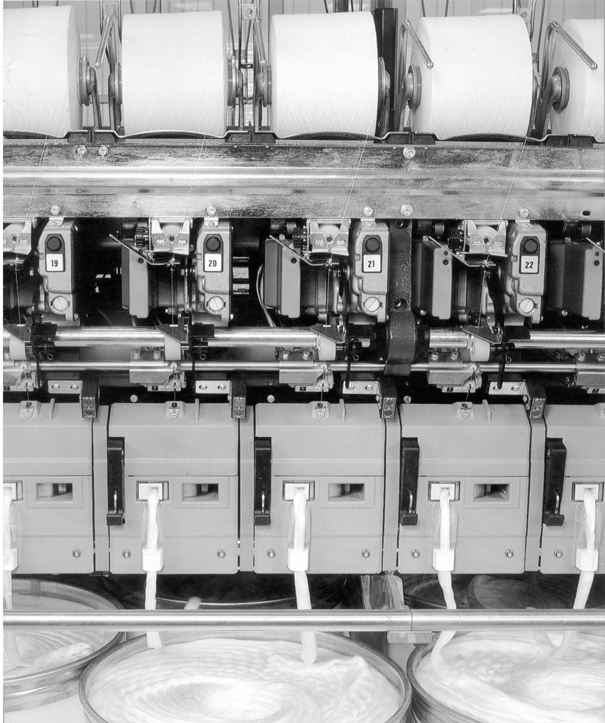
Fig. 54 Rotor spinning frame
