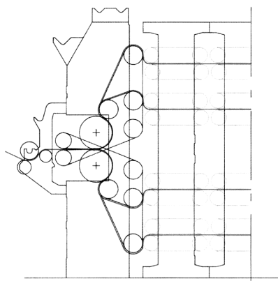
Fig. 86 Divider
