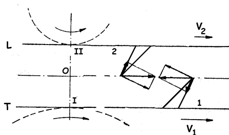
Fig. 135 Carding action
