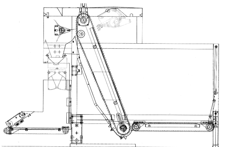
Fig. 143 – Gravimetric feeder
